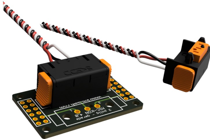
Abb. 1: Direktsteck- Technologie (Steckverbindersockel entfällt)
